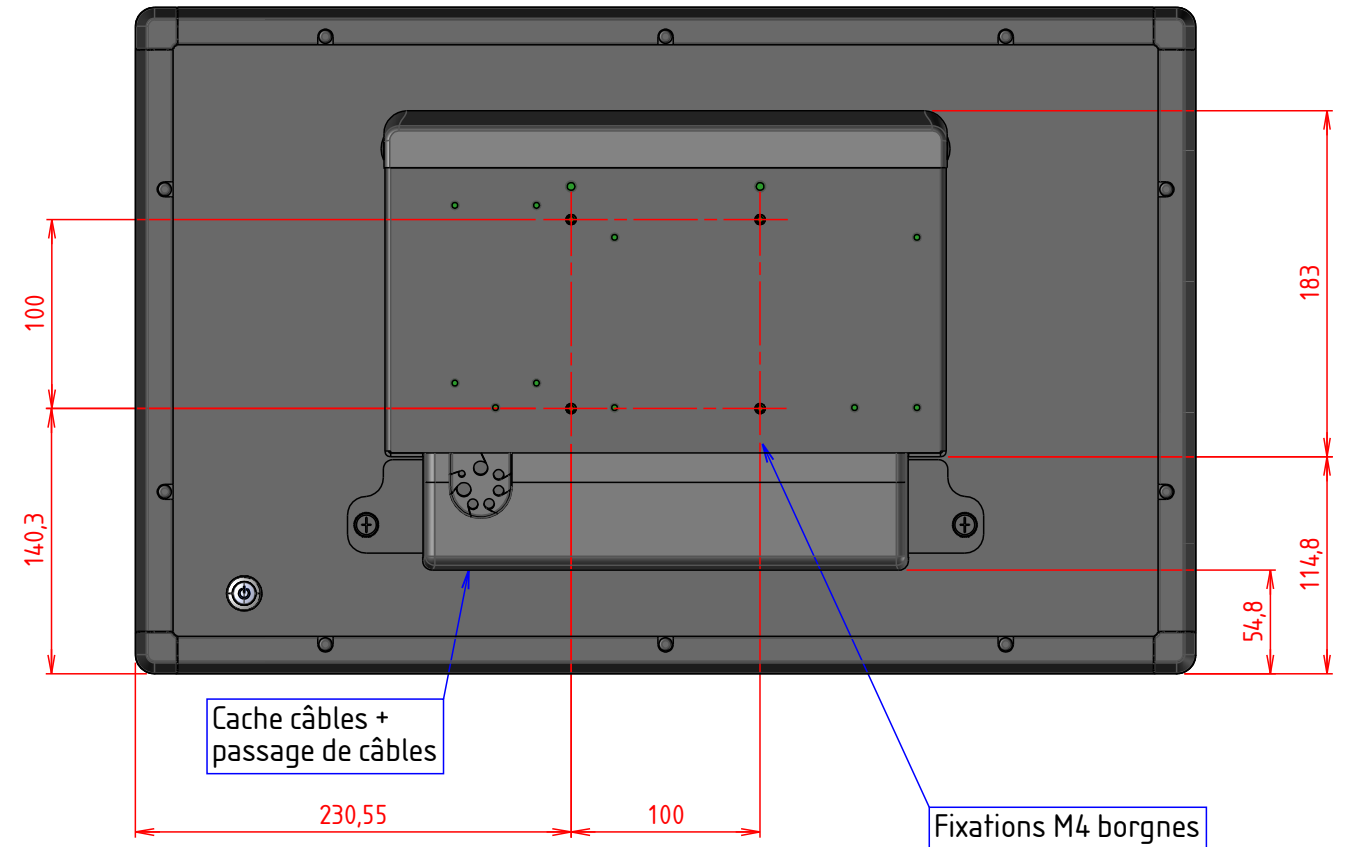
VUE ARRIERE
