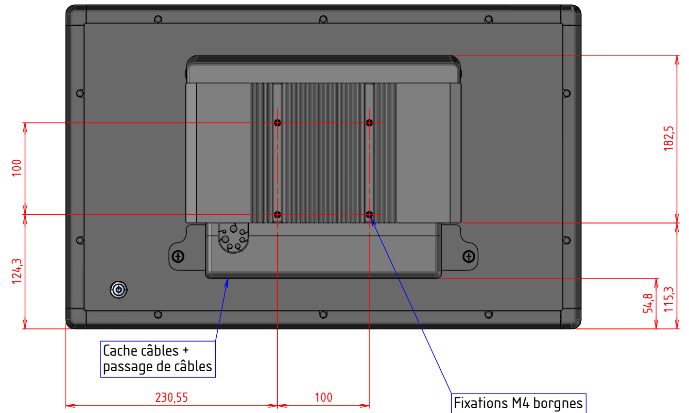
VUE ARRIERE
