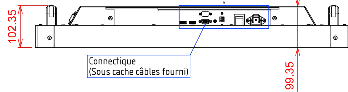
VUE DE DESSOUS
