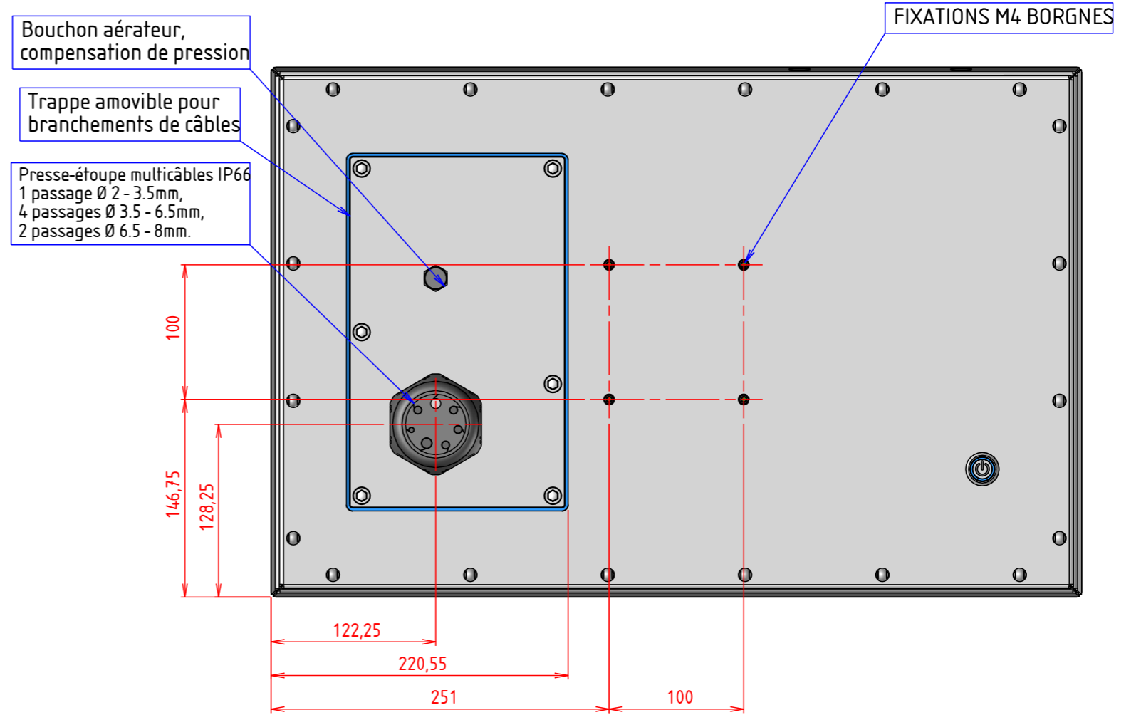
VUE ARRIERE
