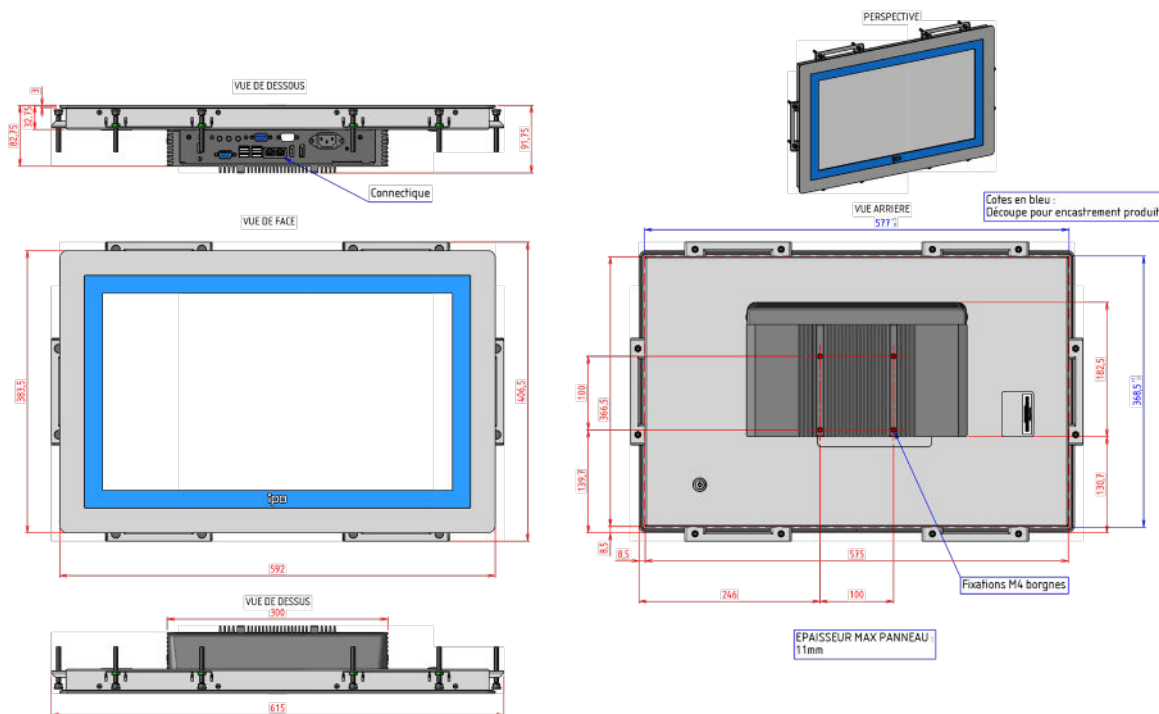
Plan de la version avec Dalle CP
