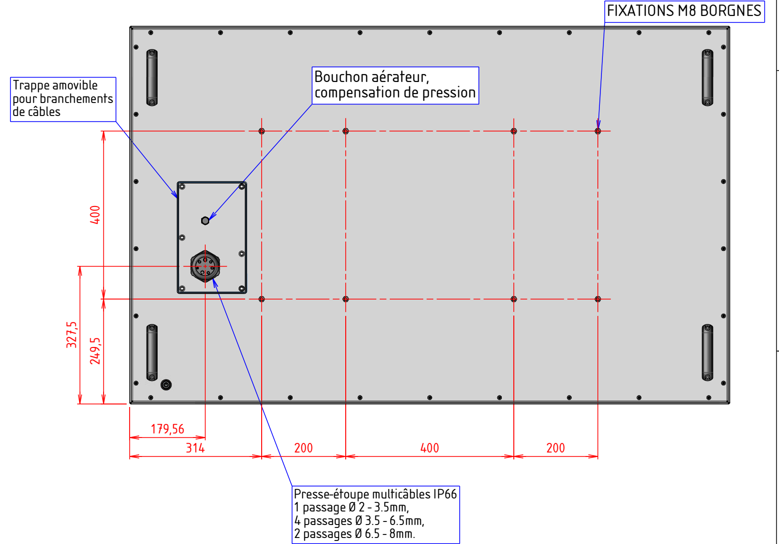
VUE ARRIERE
