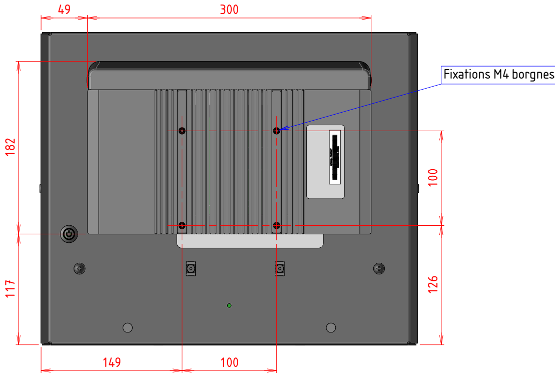
VUE ARRIERE
