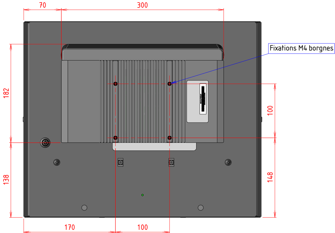
VUE ARRIERE
