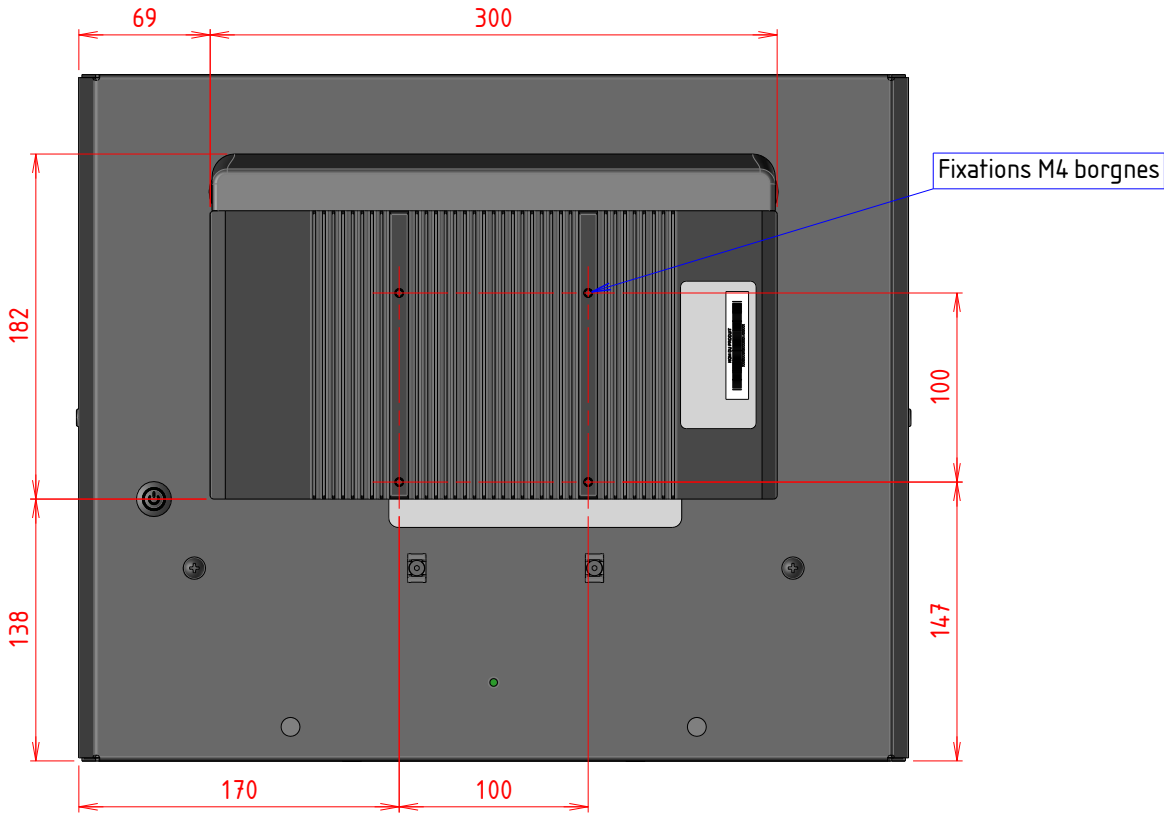
VUE ARRIERE
