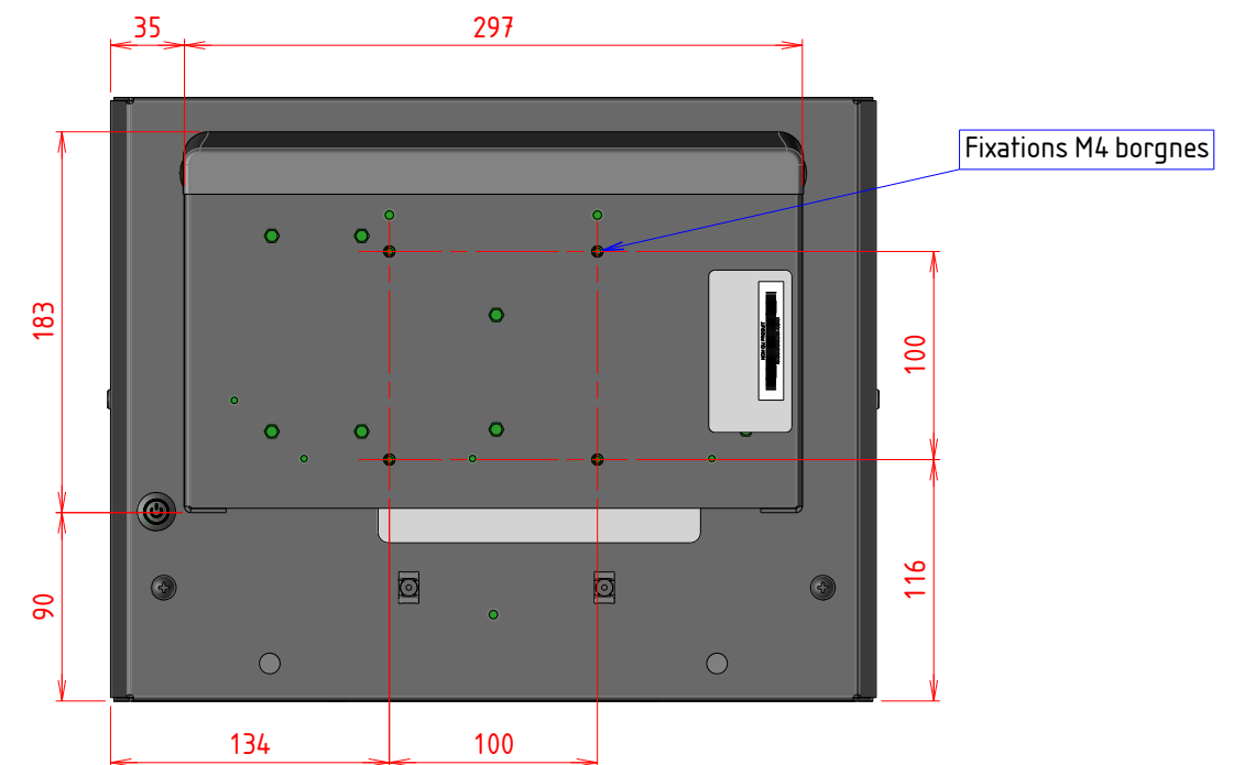
VUE ARRIERE
