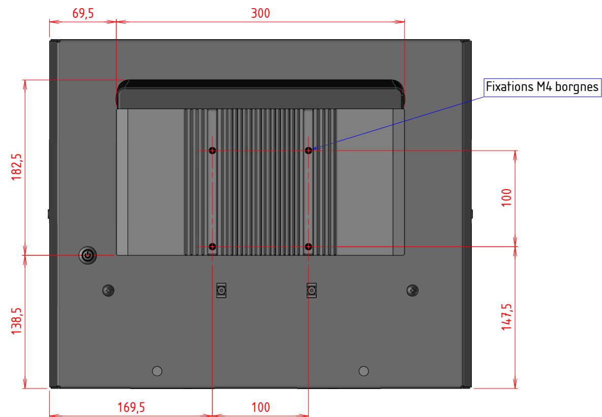
VUE ARRIERE
