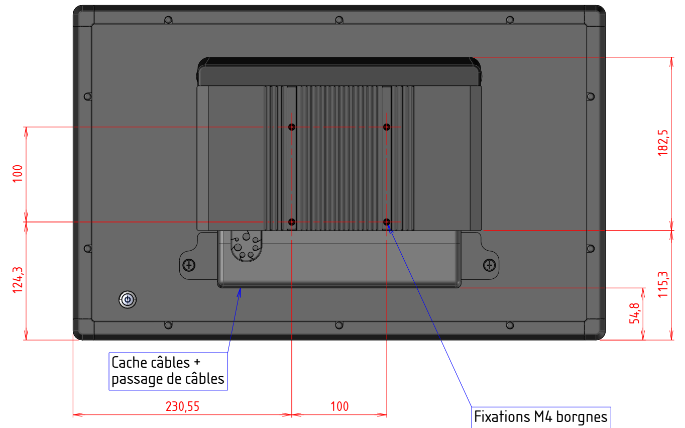
VUE ARRIERE
