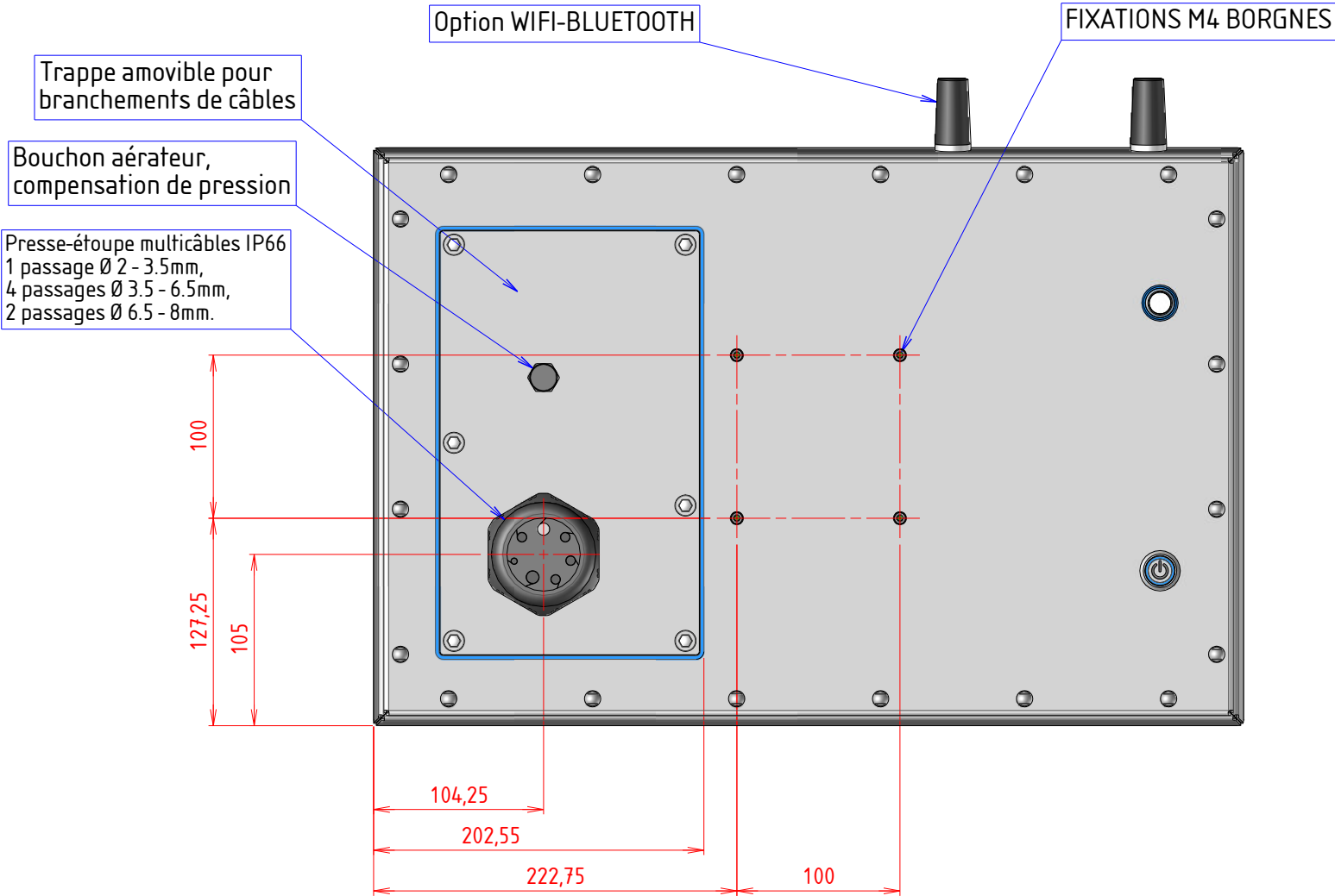
VUE ARRIERE
